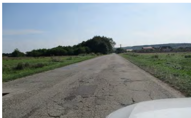
Degradări ale părții carosabile pe DJ 664A, km 16+020- km 18+920
